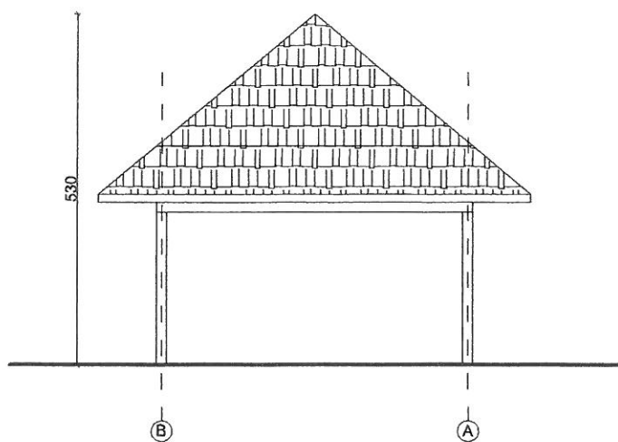
ELEWACJA PÓŁNOCNO - ZACHODNIA / ELEWACJA POŁUDNIOWO - WSCHODNIA
