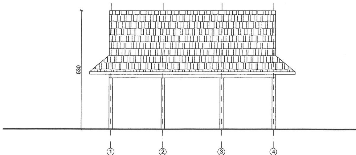
ELEWACJA PÓŁNOCNO - WSCHODNIA / ELEWACJA POŁUDNIOWO - ZACHODNIA
